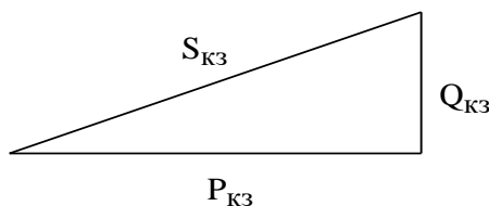
Рисунок 3 – Треугольник мощностей короткого замыкания трансформатора
