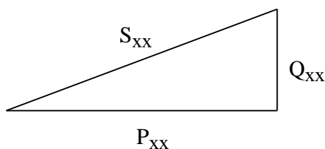
Рисунок 4 – Треугольник мощностей холостого хода трансформатора
